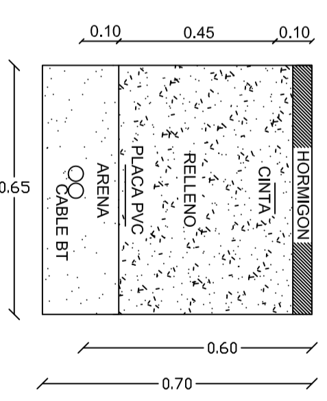
ZANUA BT EN VIAL
