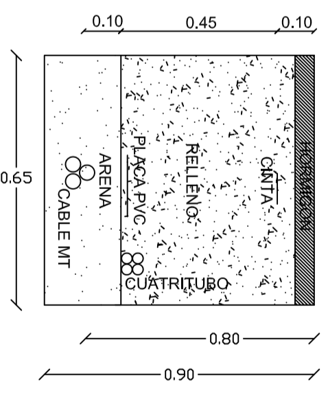
ZANUA MT EN VIAL
