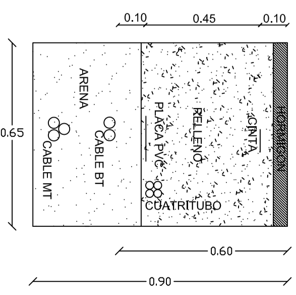
ZANUA MT/BT EN VIAL
