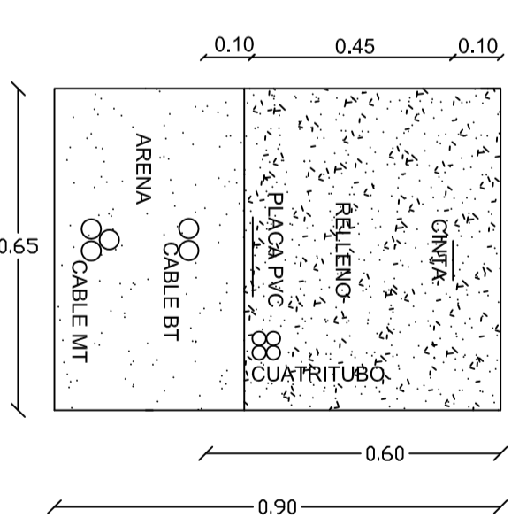
ZANUA MT/BT FUERA VIAL
