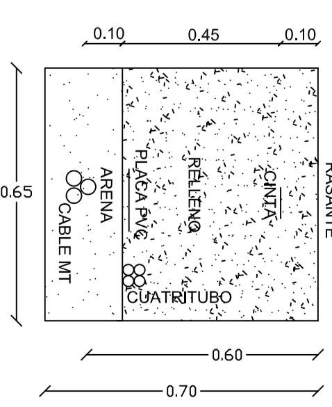
ZANUA MT FUERA VIAL
