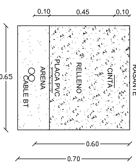
ZANUA BT FUERA VIAL
